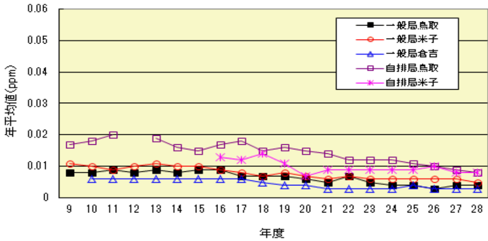
図3 二酸化窒素の年平均値
