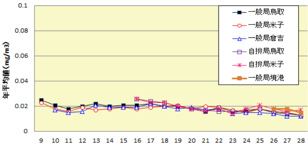
図2 浮遊粒子状物質の年平均値
