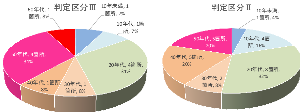
図5.2 判定区分別トンネル建設年代分け
