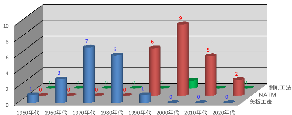
図3.3 建設年代別道路トンネル箇所数
