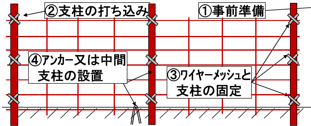
1枚のワイヤーメッシュ(長さ2.0m)の間に「アンカー」又は「中間支柱」を設置
