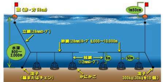
籠数は、1連に180個取り付けれる。
