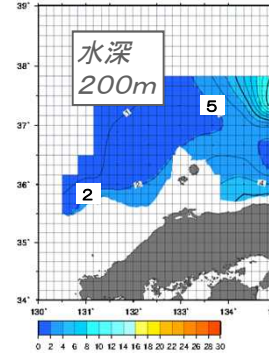
兵庫県沖の北緯38°00'付近に暖水塊が分布しています。
