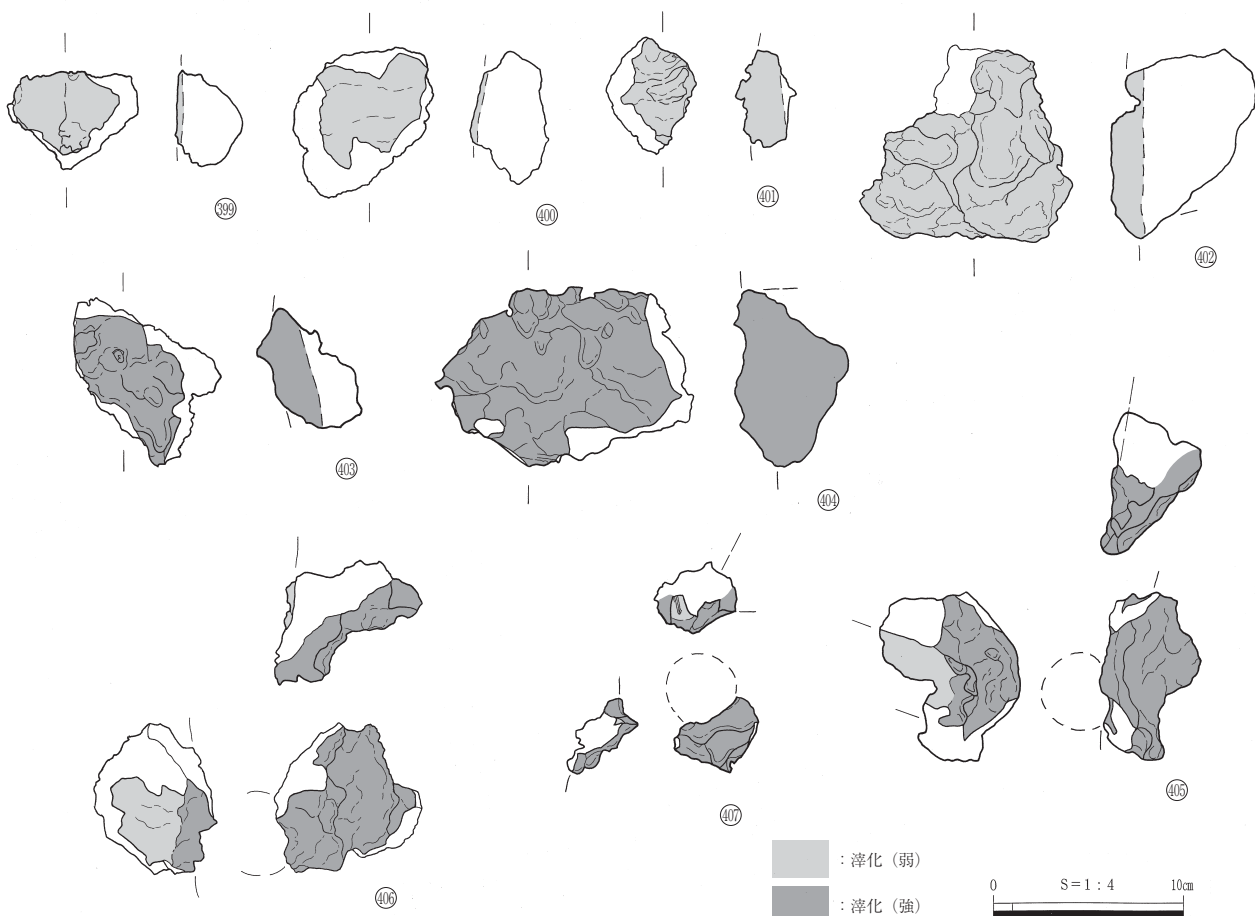
第204図 表土出土製鉄関連遺物(1)
