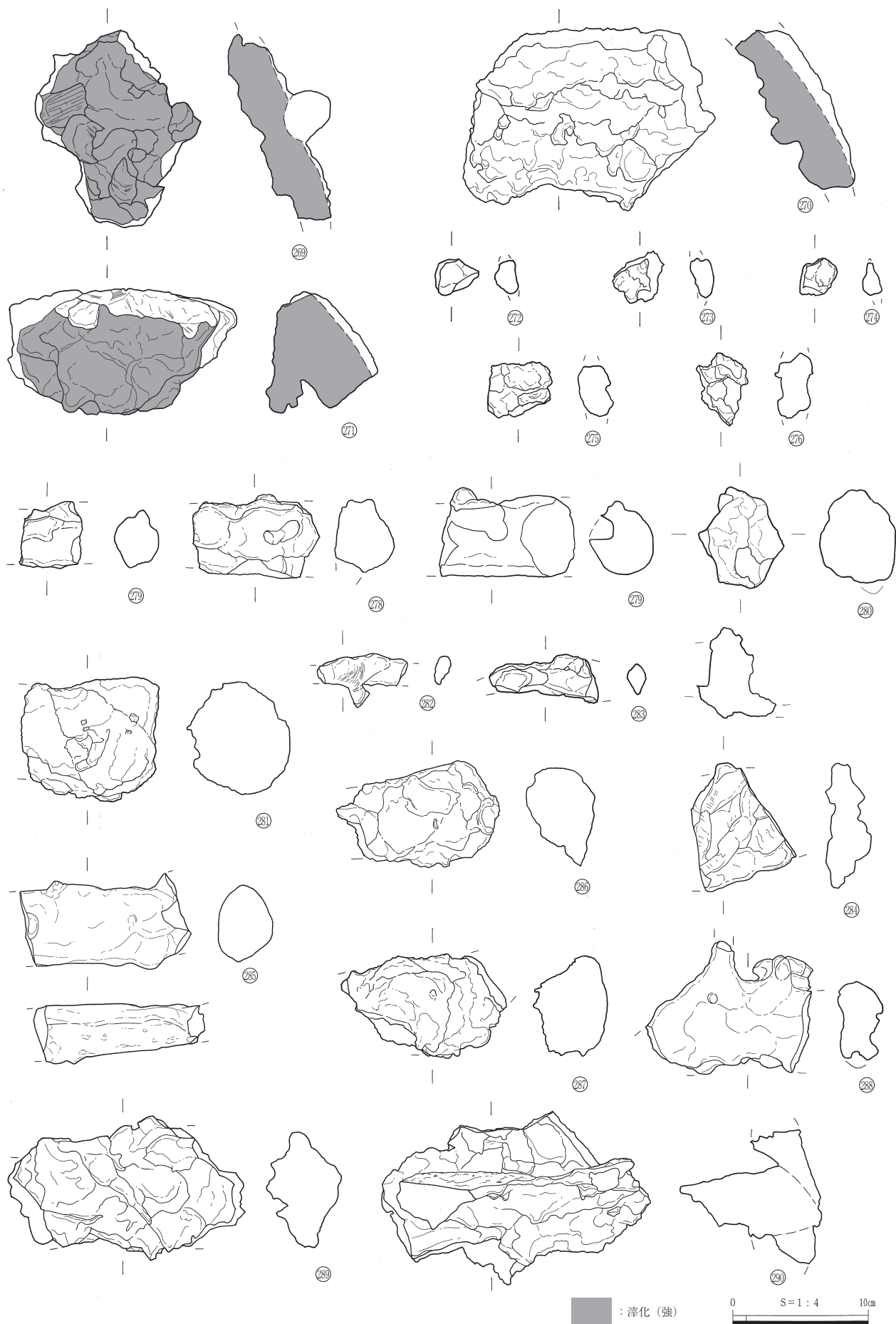
第193図 排滓場1出土製鉄関連遺物(4)
