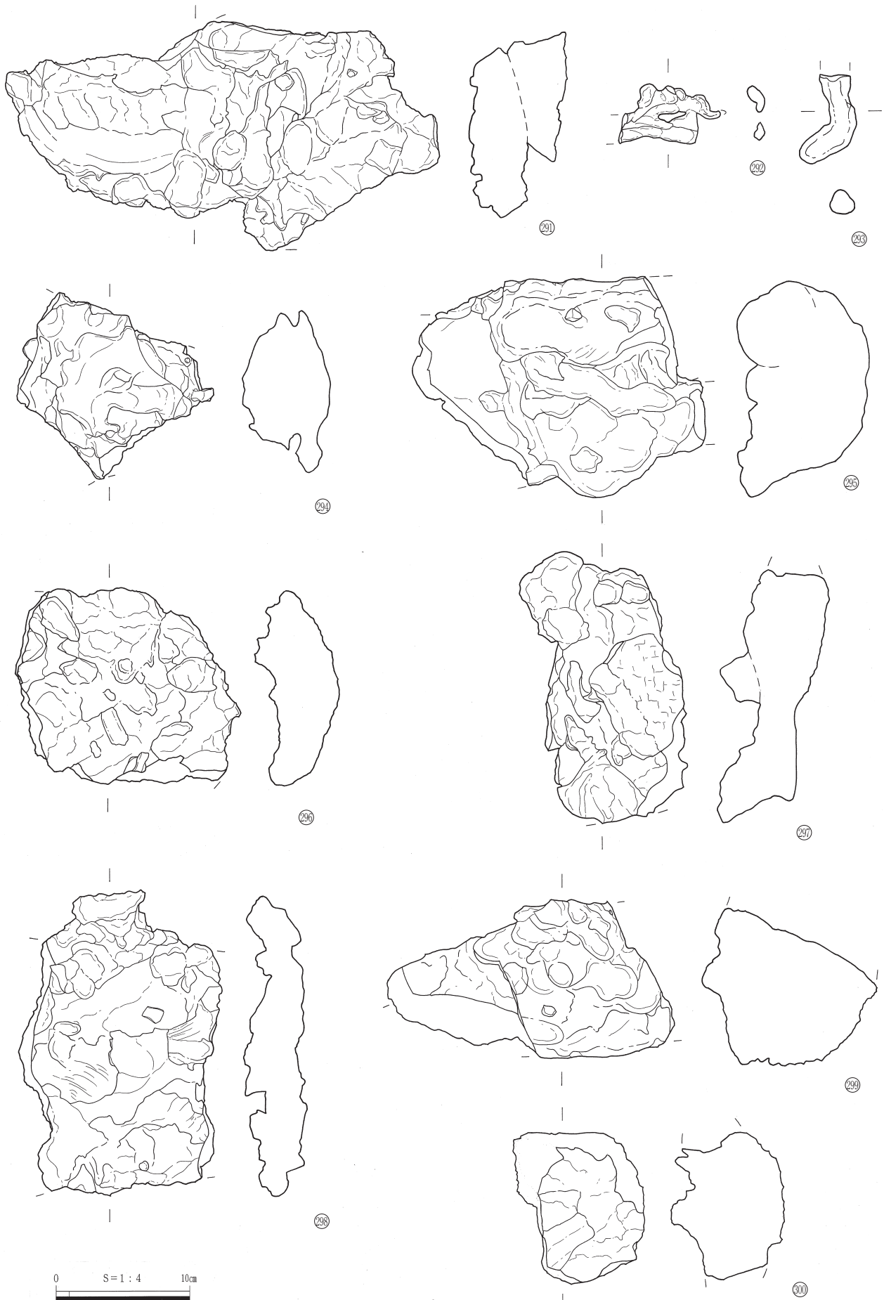
第194図 排滓場1出土製鉄関連遺物(5)
