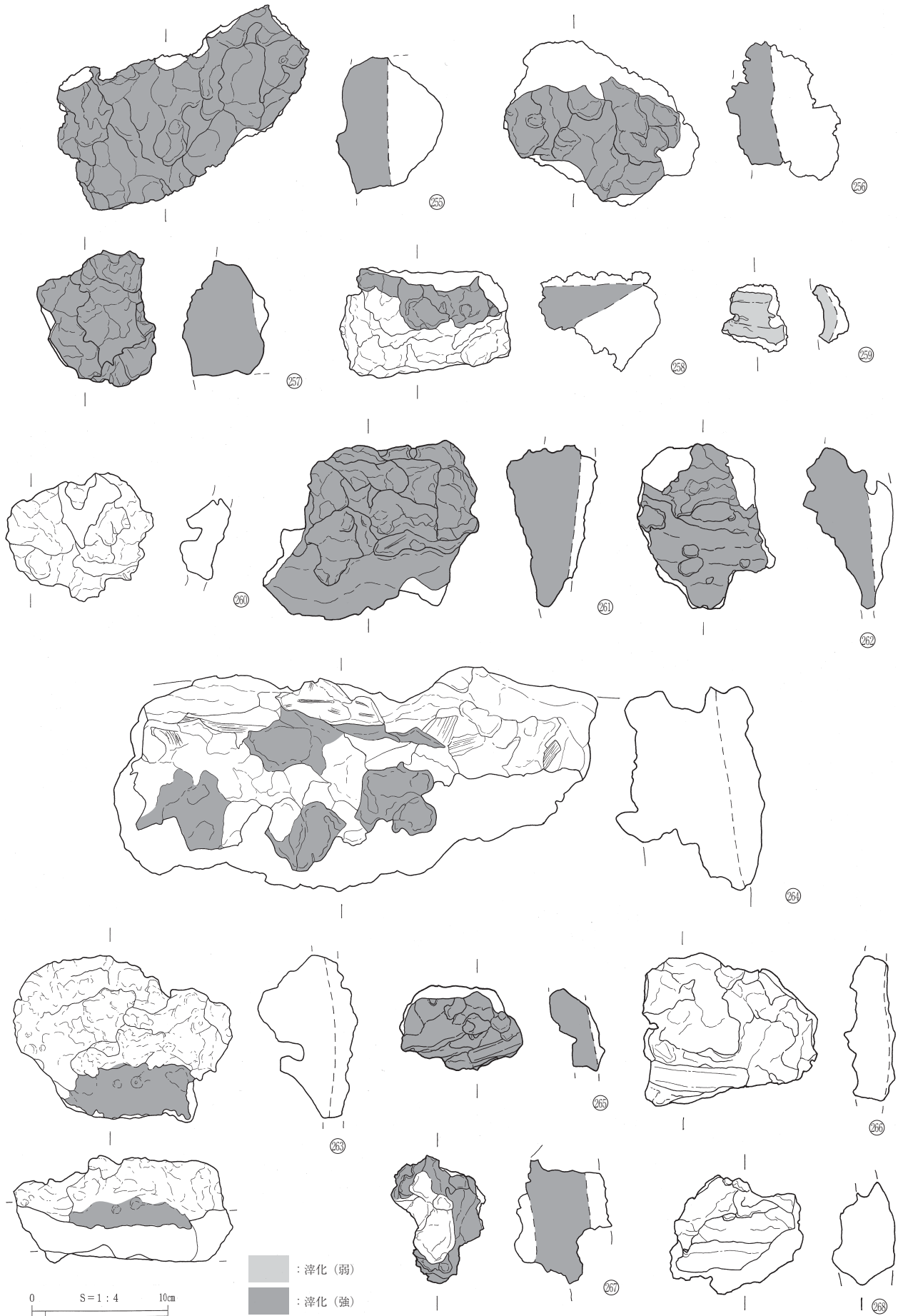
第192図 排滓場1出土製鉄関連遺物(3)
