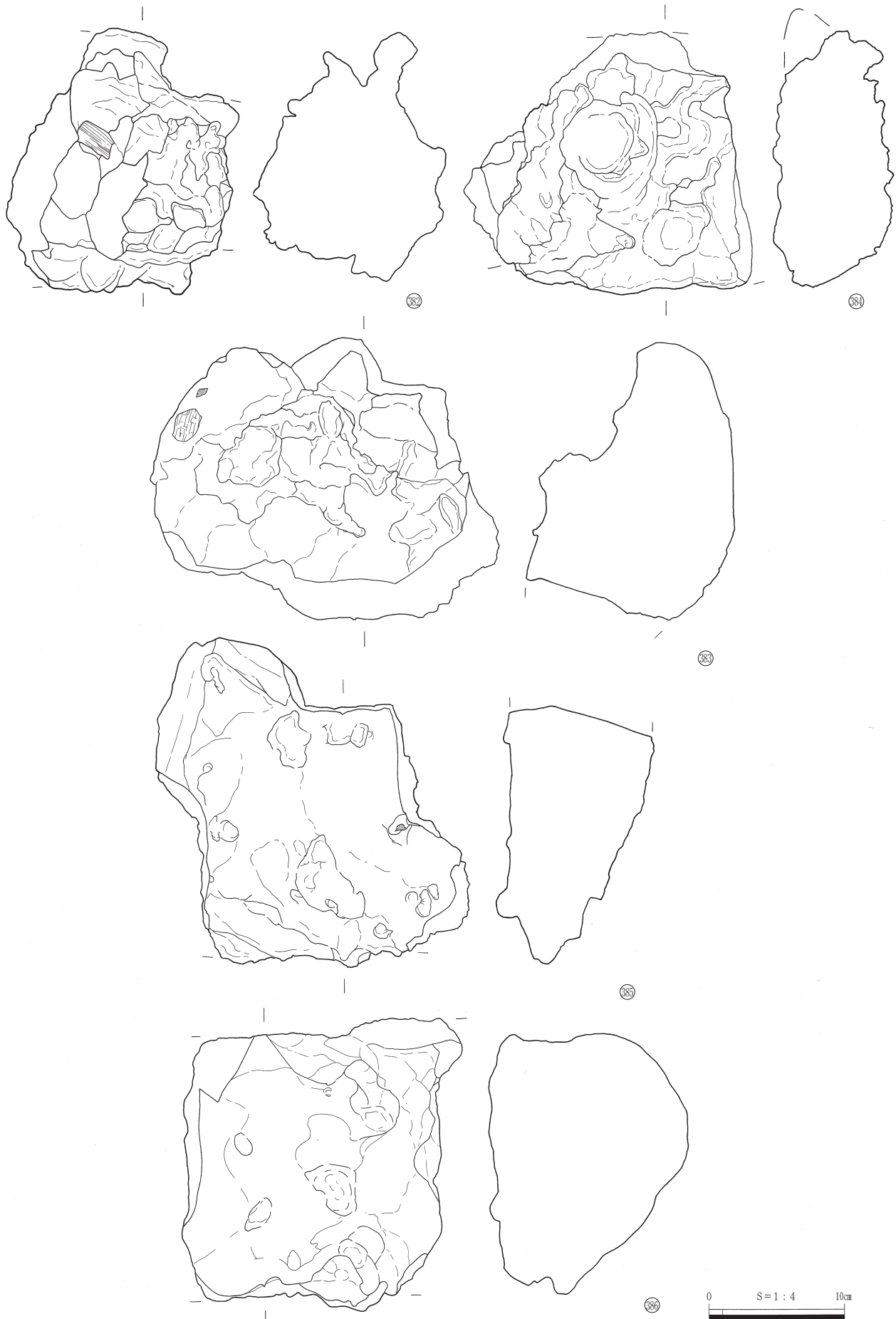
第201図 排滓場2出土製鉄関連遺物(6)
