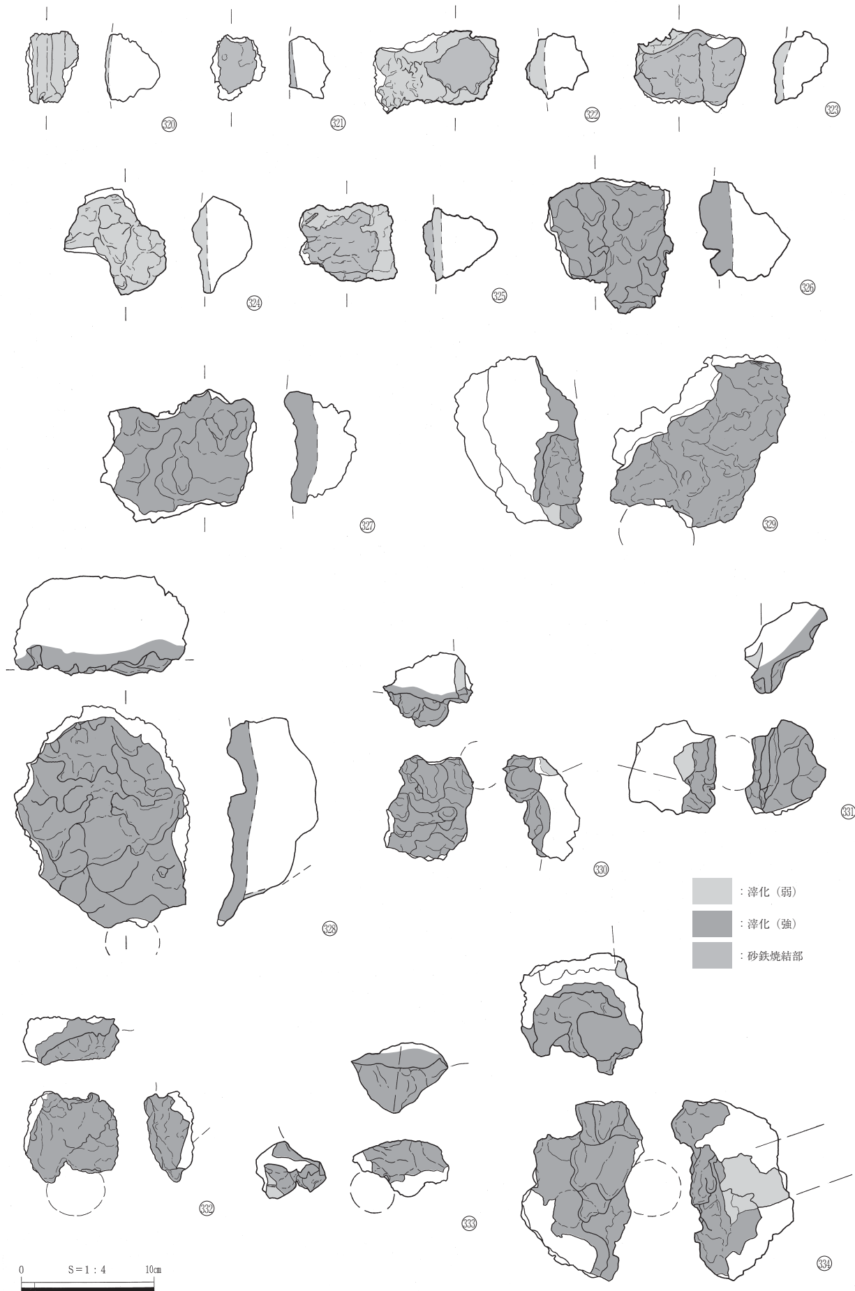
第196図 排滓場2出土製鉄関連遺物(1)
