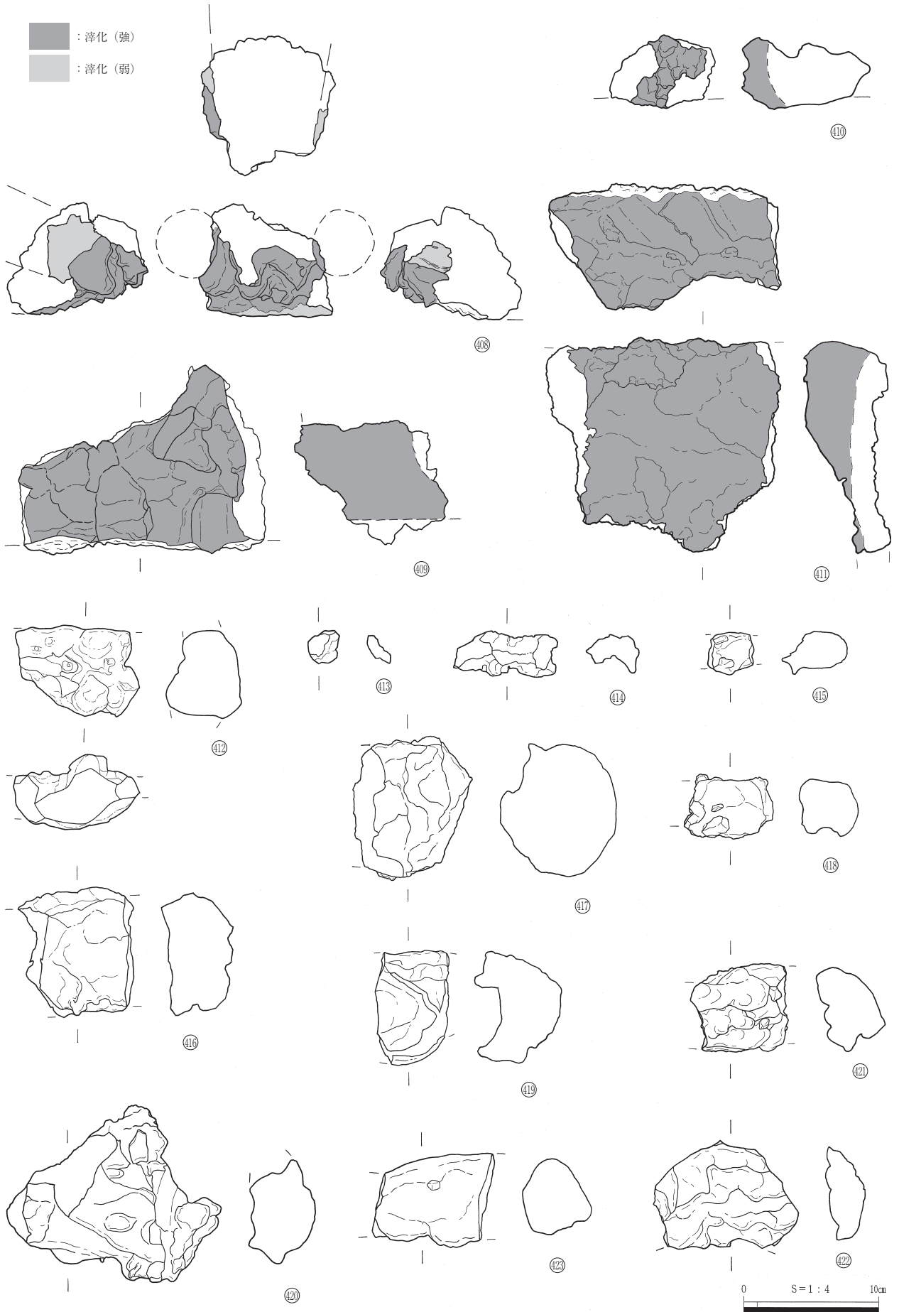
第205図 表土出土製鉄関連遺物(2)
