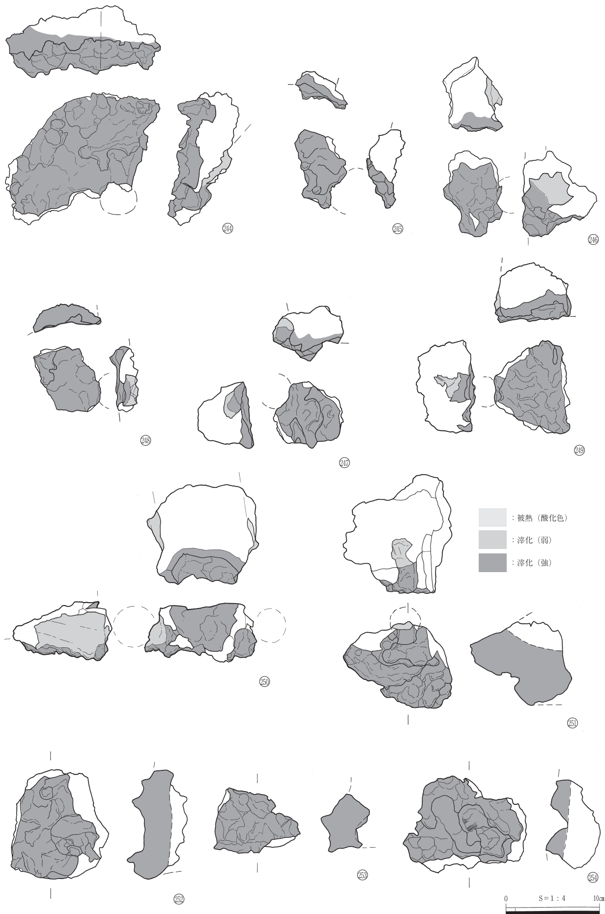
第191図 排滓場1出土製鉄関連遺物(2)
