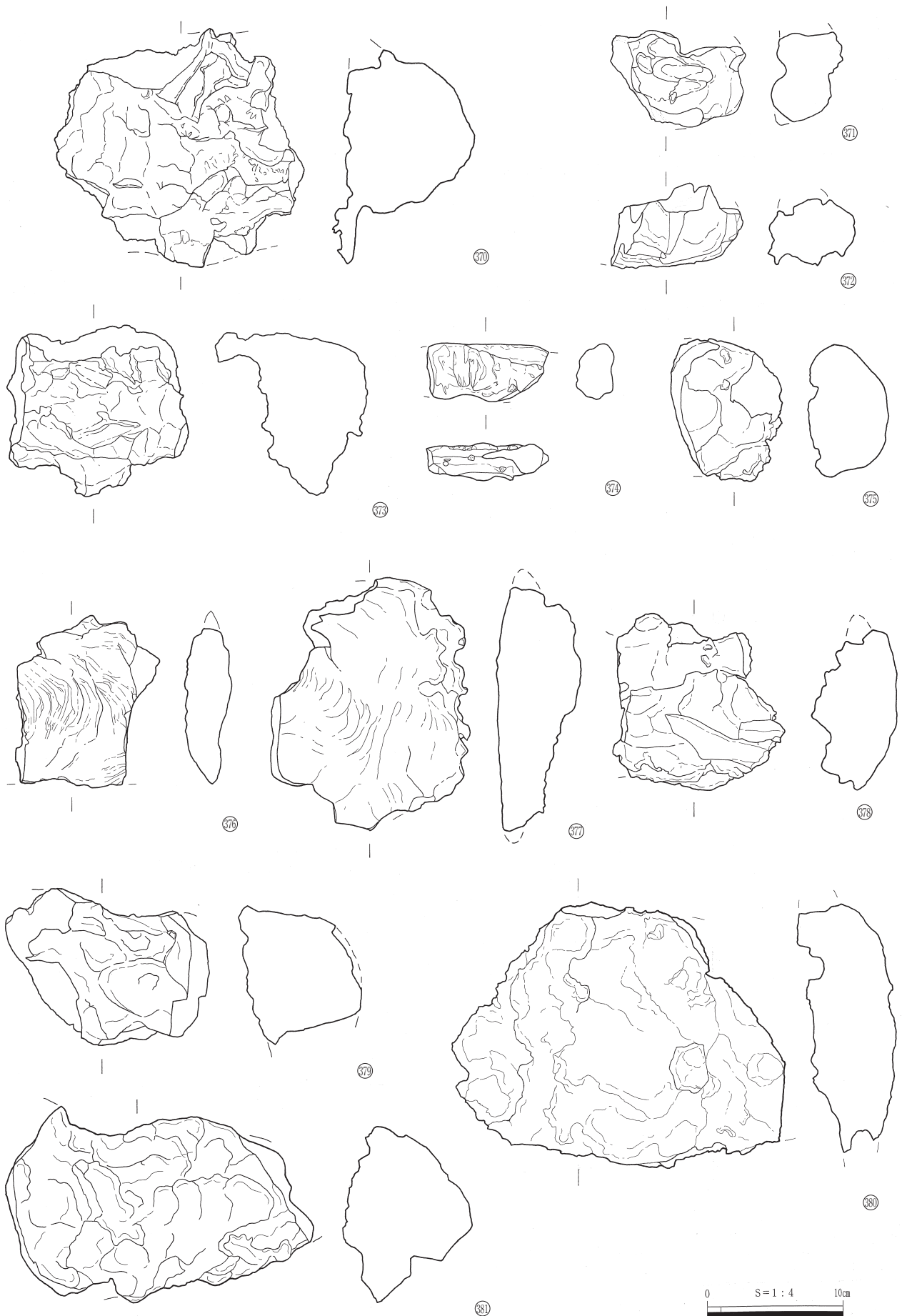
第200図 排滓場2出土製鉄関連遺物(5)
