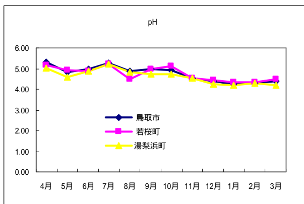
図1 平成18年度における pH の経月変化
