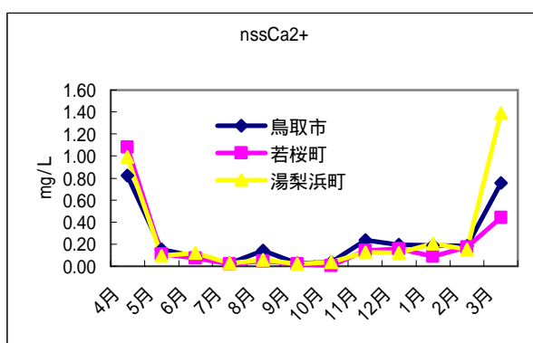
図4 平成18年度における nss-Ca 2+ 濃度の経月変化
