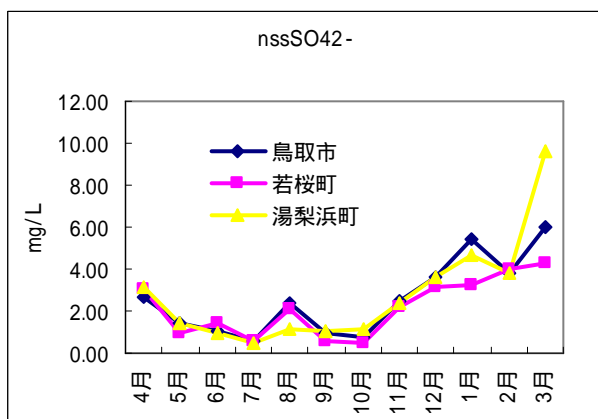
図2 平成18年度における nss-SO 4 2- 濃度の経月変化
