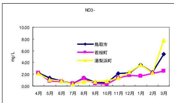
図3 平成18年度における NO 3 - 濃度の経月変化
