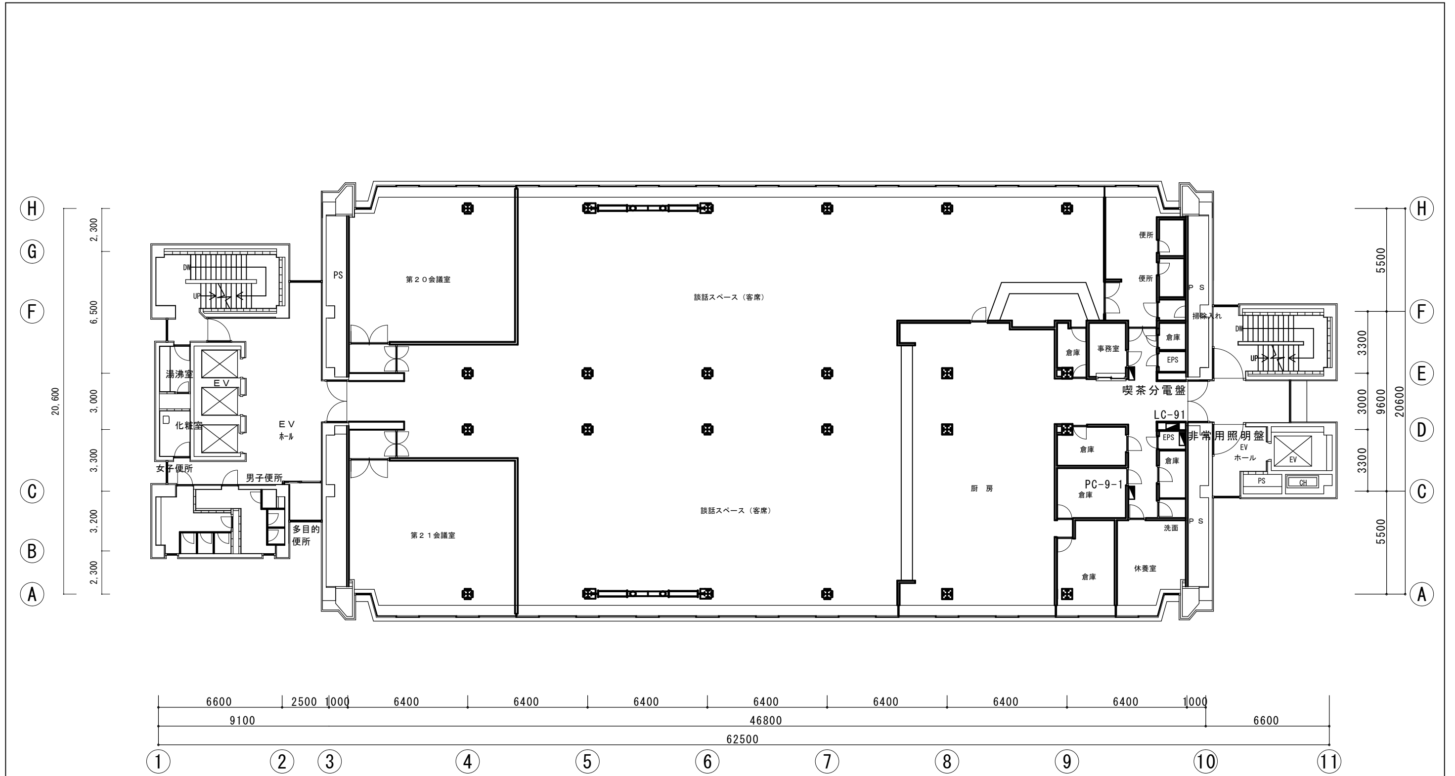
第二庁舎 9階平面図 1/200
