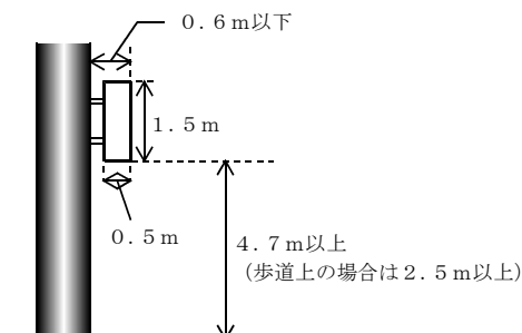
【図8-1】電柱に添加する場合
