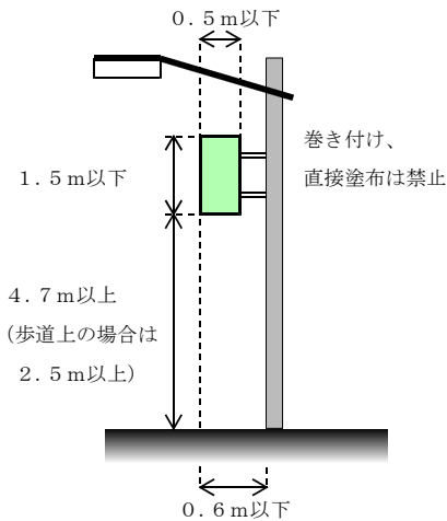
【図9】街灯柱
