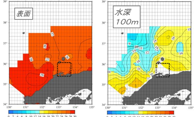
随崎海峡と鳥取県沖(点線範囲内)の平均水温は27.6℃(28.2～26.7℃)を示しています。【前年差:+0.06℃、平年(直近30年)差:+1.43℃】 平均水温は17.6℃(17.1～18.3℃)を示しています。【前年差:+0.13℃、平年(直近30年)差:+1.53℃】
