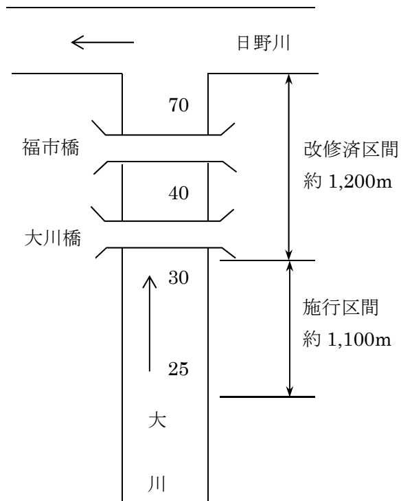
図 4.1.3 大川整備計画流量
