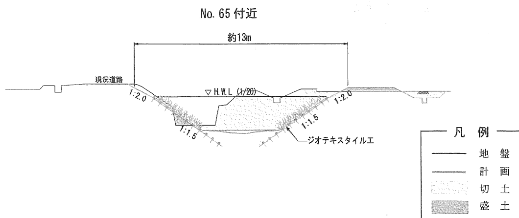
図 4.1.4 大川代表断面図
