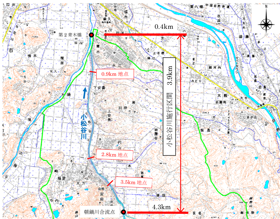
図 4.1.5 小松谷川整備箇所位置図
