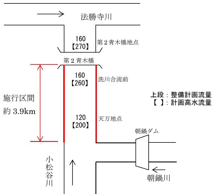
図 4.1.6 小松谷川計画高水流量配分図
