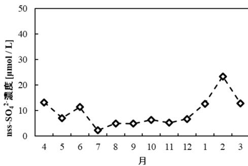
図5 降水中 nss-SO 4 2- 濃度の経月変化
