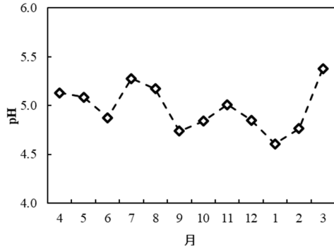
図2 降水 pH の経月変化
