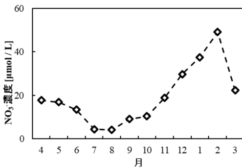
図4 降水中 NO 3 - 濃度の経月変化
