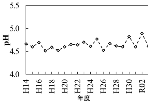
図3 降水 pH (年加重平均値) の経年変化
