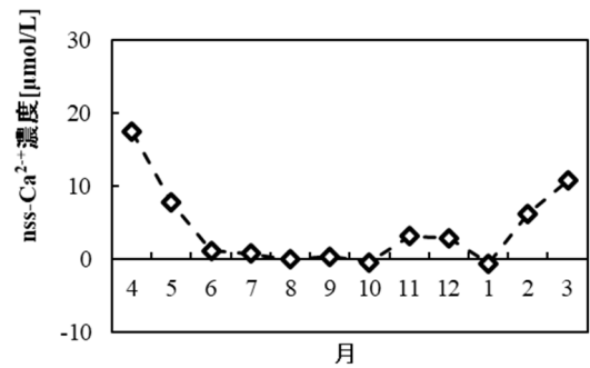
図7 降水中の nss-Ca 2+ の経月変化
