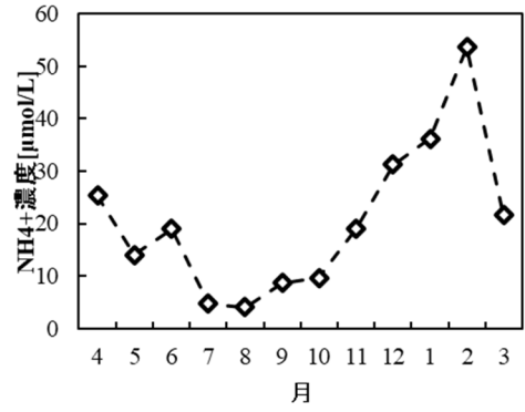
図6 降水中の NH 4 + の経月変化
