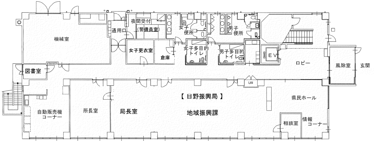
1階平面図
