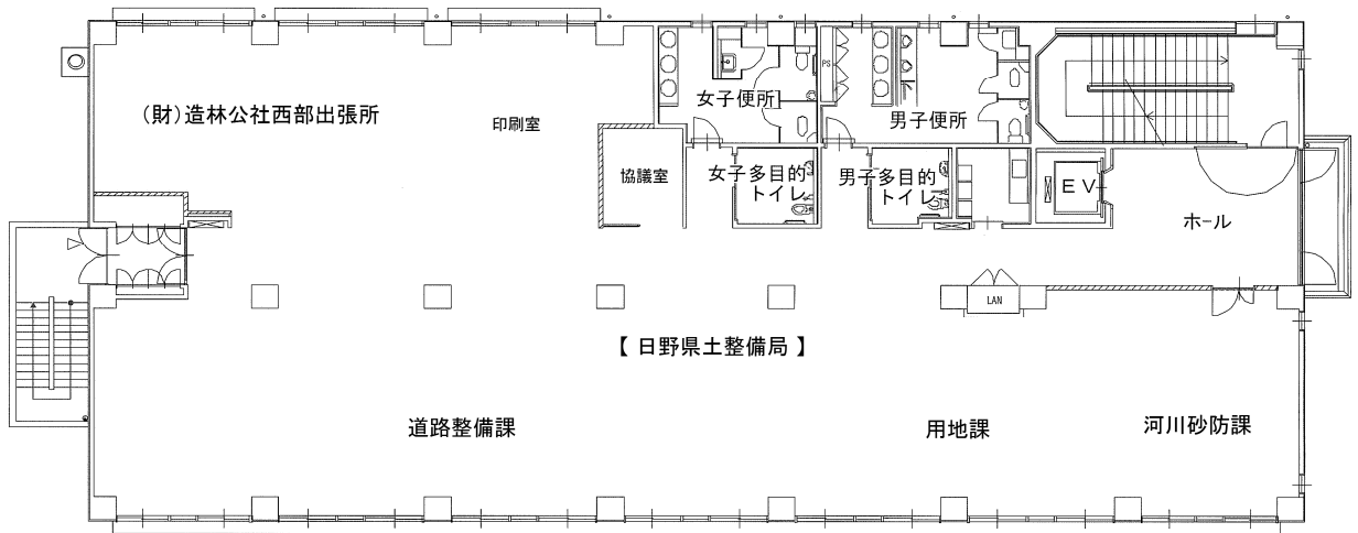
3階平面図
