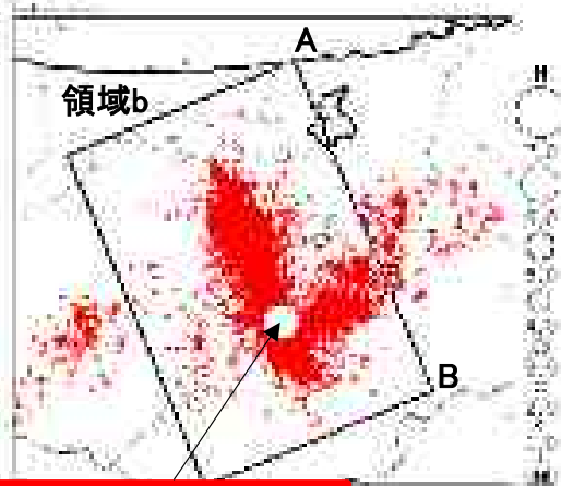
震央分布図
