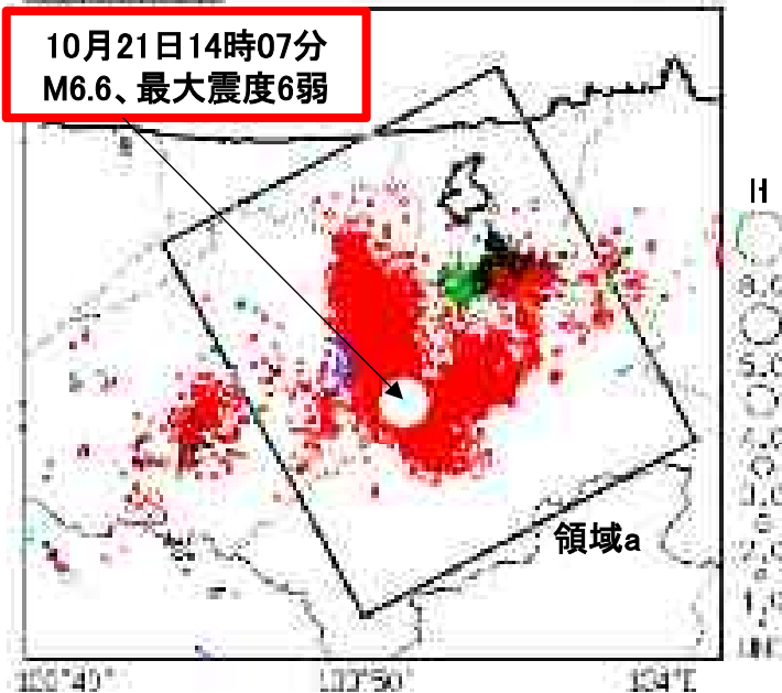
震央分布図
