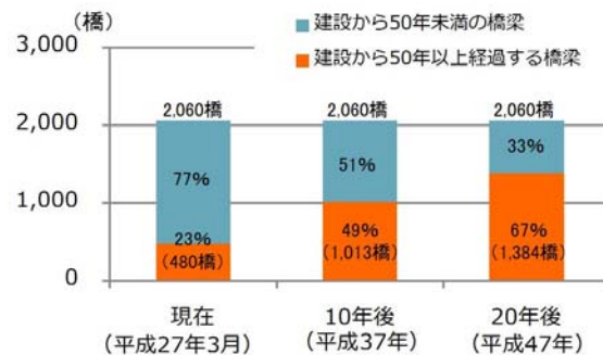
図 4.2 橋梁の老朽化推移予測(鳥取県) 出典：鳥取県道路橋りょう長寿命化計画
