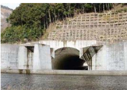
河川トンネル（市瀬トンネル）
