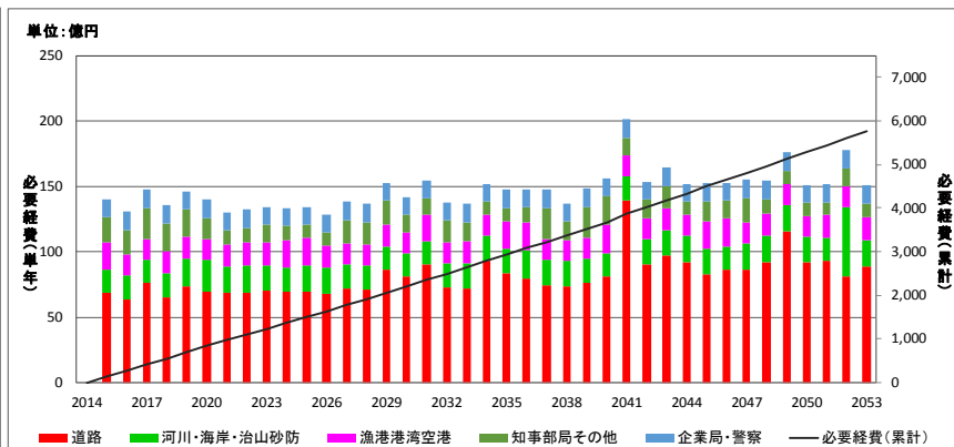
図 6.7 鳥取県の土木インフラの維持管理・更新費(生涯経費推計)
